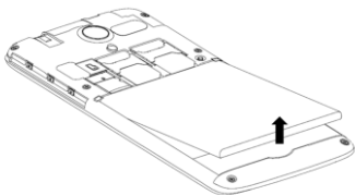
图 2 拆卸电池
